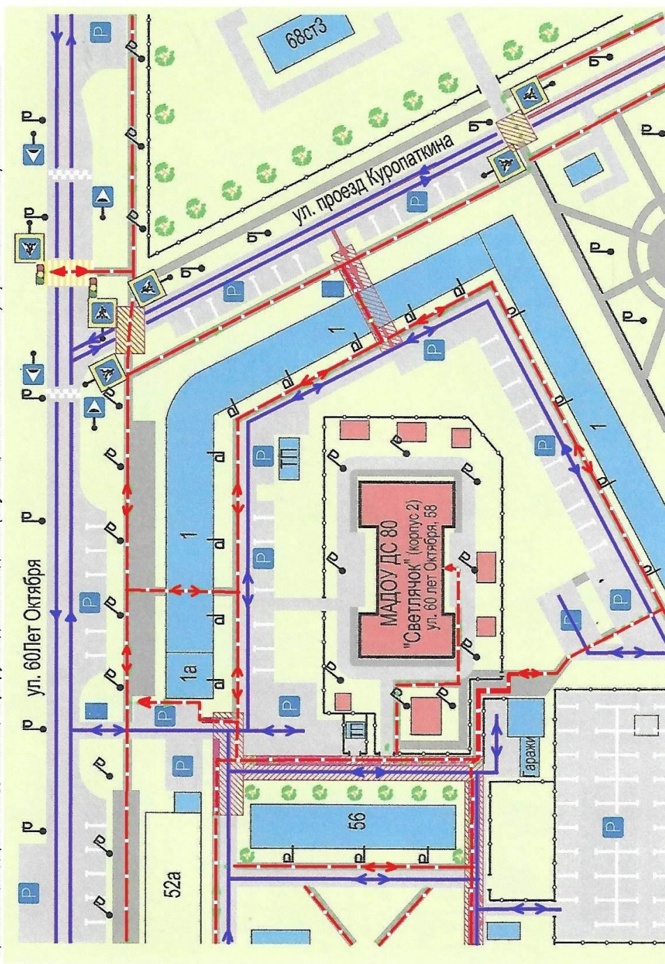
Схема организации дорожного движения в непосредственной близости от образовательного учреждения с размещением соответствующих технических средств организации дорожного движения, маршрутов движения детей (обучающихся и воспитанников) и расположения парковочных мест
